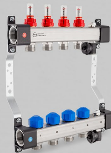
Rozdzielacze z przepływomierzami i zaworami do siłowników oraz sekcją odpowietrzającą - seria N75A
