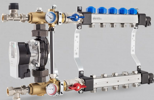
Rozdzielacze z zaworami regulacyjnymi i zaworami do siłowników oraz układem mieszającym z pompą elektroniczną - seria N73E
