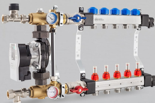
Rozdzielacze z przepływomierzami i zaworami do siłowników oraz układem mieszającym z pompą elektroniczną - seria N77E
