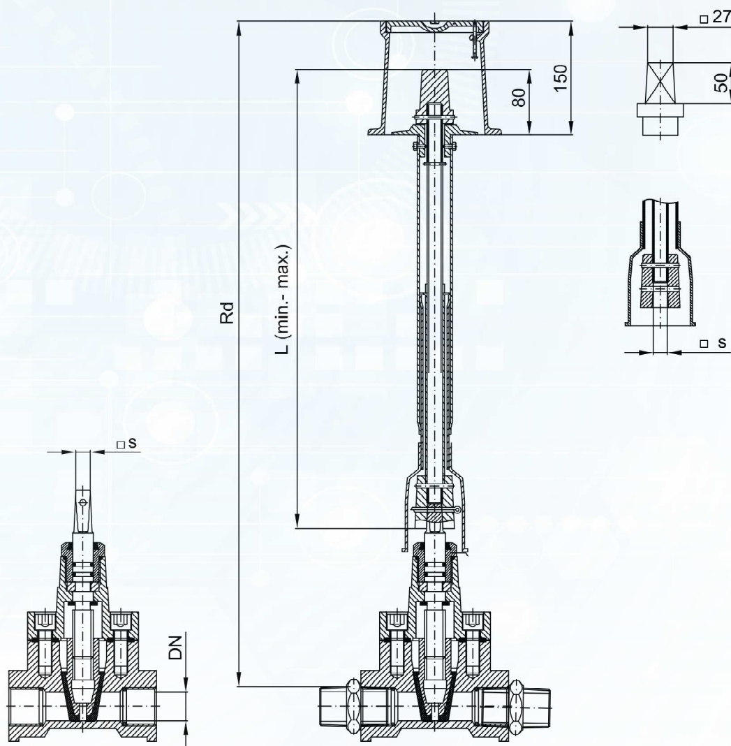
Skrzynka uliczna - wysokość 150 mm.
