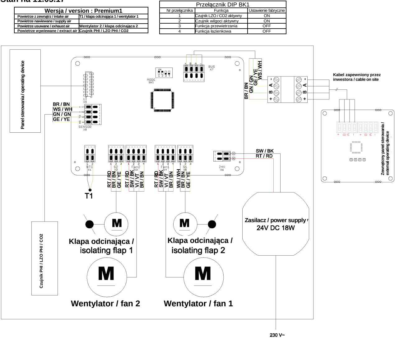
Schemat zacisków RC CA 70 Premium 1 Stan na 11.05.17
