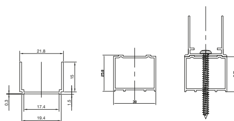
Capital profil poszerzający do kabin ze ścianką stałą, do drzwi ze ścianką stałą i ścianek stałych: AM43..., AM44..., AM46..., AM48195020 Szerokość 20 mm
