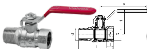
Kurek kulowy ONYX z dławikiem, nakrętno-wkrętny z dźwignią stalową
