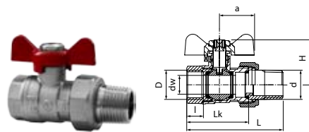
Kurek kulowy ONYX z dławikiem, z półśrubunkiem z motylikiem aluminiowym
