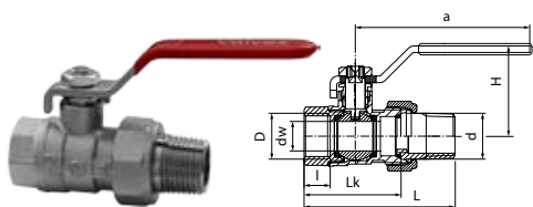
Kurek kulowy ONYX z dławikiem, z półśrubunkiem z dźwignią stalową
