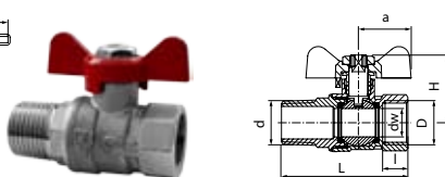
Kurek kulowy ONYX z dławikiem, nakrętno-wkrętny z motylikiem aluminiowym
