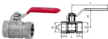
Kurek kulowy ONYX z dławikiem, nakrętno-nakrętny z dźwignią stalową
