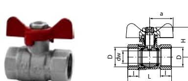
Kurek kulowy ONYX z dławikiem, nakrętno-nakrętny z motylikiem aluminiowym
