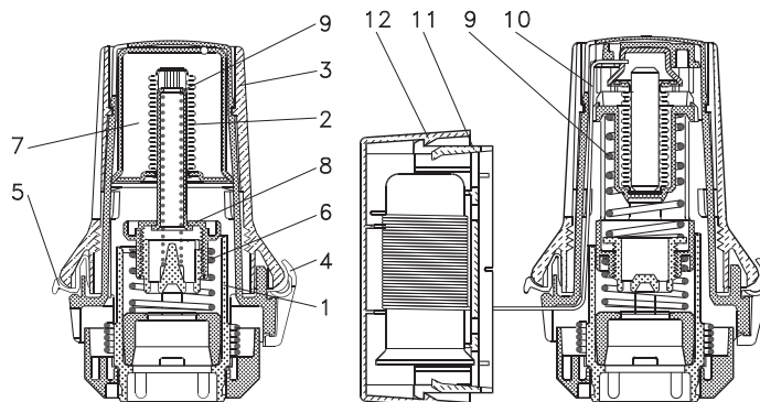
Czujnik wbudowany
