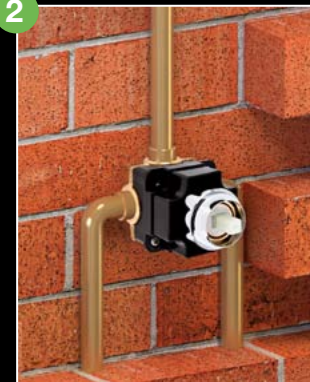
Zainstalowanie elementu podtynkowego.
