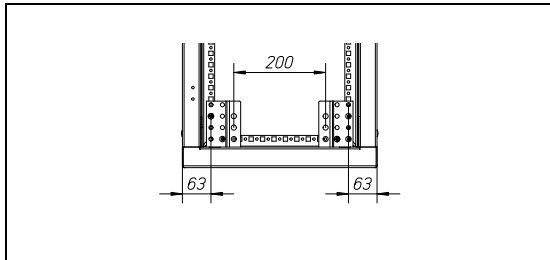
Width 600mm
