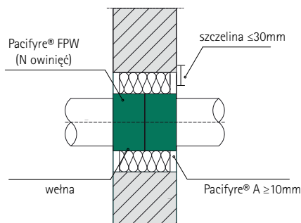
aplikacja dwustronna w ścianach
