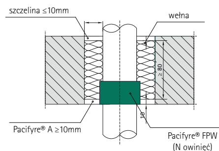
aplikacja jednostronna w stropach
