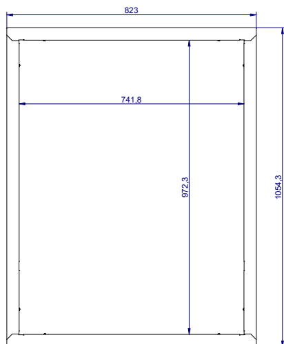
Ramki do szaf 780x1010
