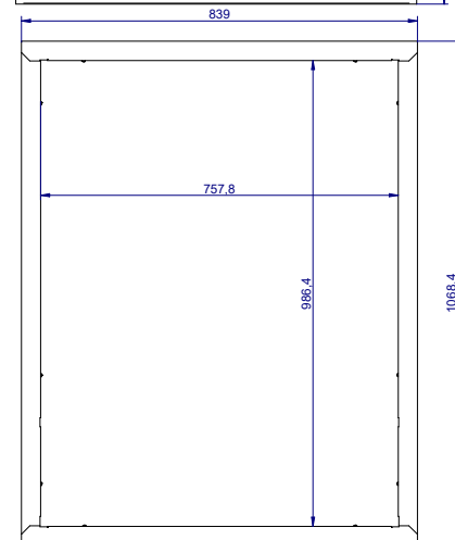
Ramki do szaf 795x1025
