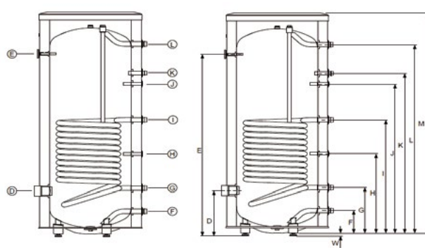
ZASOBNIK Z JEDNĄ WĘŻOWNICĄ MEGA 300.81.ONN
