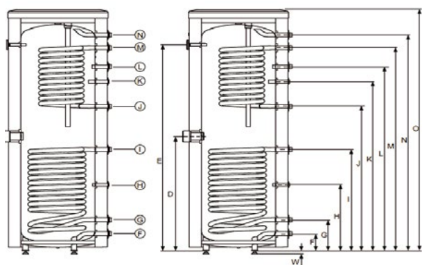
ZASOBNIK Z DWIEMA WĘŻOWNICAMI MEGA 220.82.ONN
