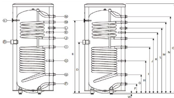
ZASOBNIK Z DWIEMA WĘŻOWNICAMI MEGA 300.82.ONN
